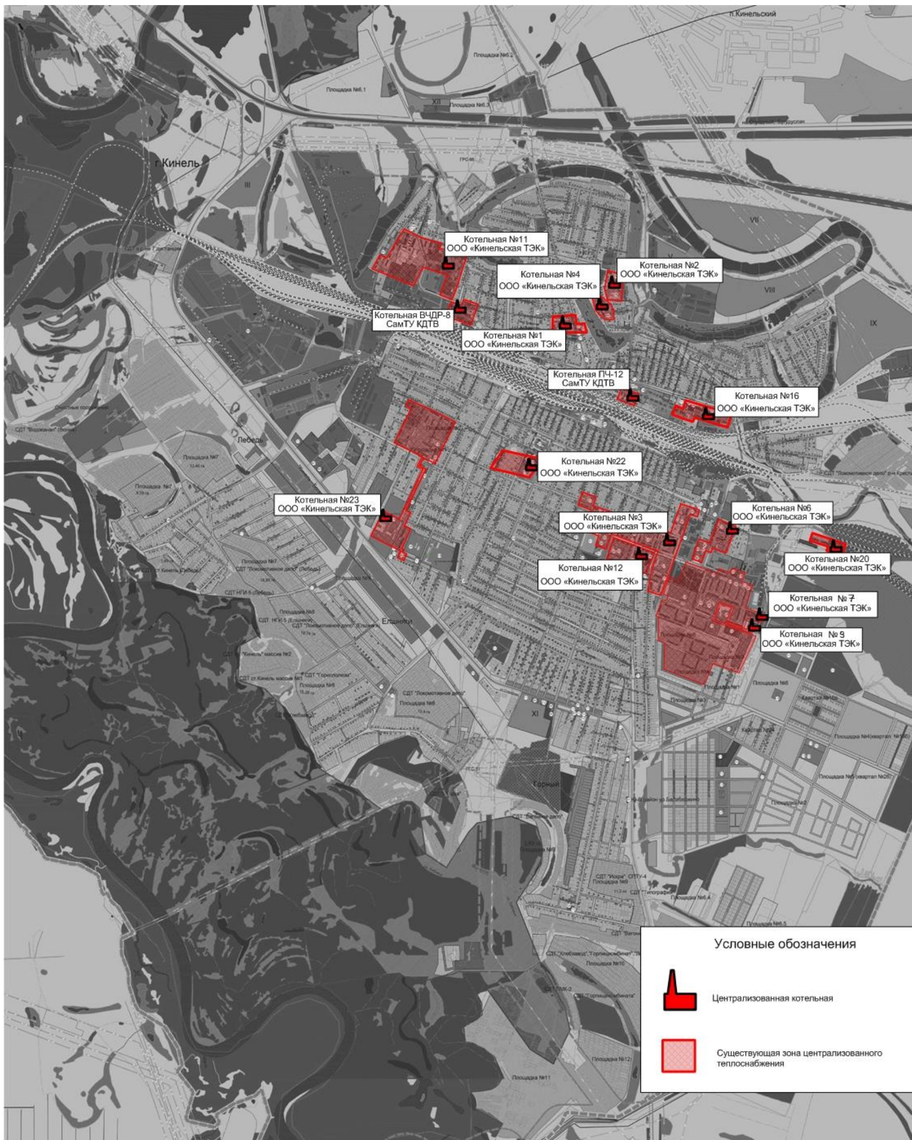
Рисунок 1.1.1.1– Зона действия централизованных систем теплоснабжения г. Кинель
